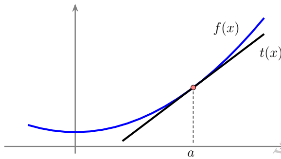
Figura 1.1.2: Significado geométrico de la derivada: f'(a) es la pendiente de la recta t(x) tangente (ver la ecuación (1.1.1)) a la curva definida por la función f(x) en el punto x = a .
