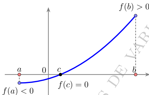
Figura 1.1.1: Esquema que ilustra el Teorema de Bolzano.
