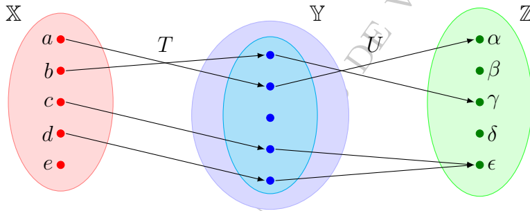
Figura 1.3.2: Composición de funciones T \circ U de T : \mathbb{X} \mapsto \mathcal{I}(T) \subset \mathbb{Y} y U : \mathcal{D}(U) \subset \mathbb{Y} \mapsto \mathbb{Z} , donde \mathcal{I}(T) \subset \mathcal{D}(U) .
