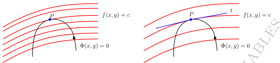
Figura 4.2.1: Curvas de nivel de f(x, y) (en rojo) y curva \Phi(x, y) = 0 (negro). En la figura de la derecha además está representada la recta tangente t (azul) en el punto P = (x_0, y_0) .
