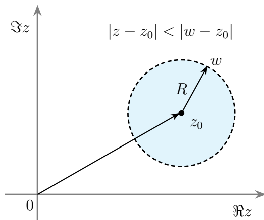
Figura 1.1: Región de convergencia de la serie \sum_{n=0}^{\infty} a_n(z - z_0)^n .
