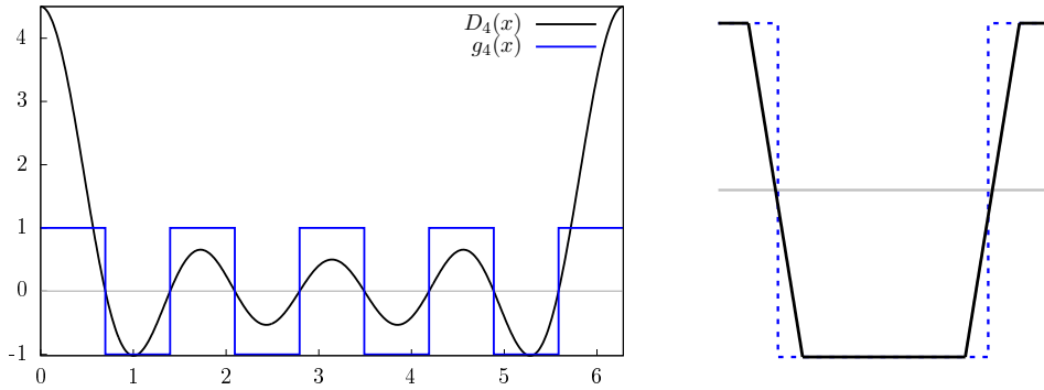
Figura 4.3: Las funciones D_4(x) y g_4(x) (izquierda) y detalle de g_k y f_k (derecha).
