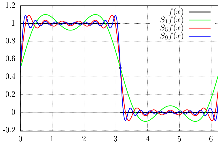
Figura 4.2: La función discontinua f y las sumas parciales de su serie de Fourier para n = 1, 5 y 9 .
